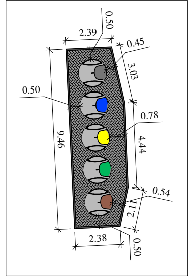
Aikštelės detalizacija
